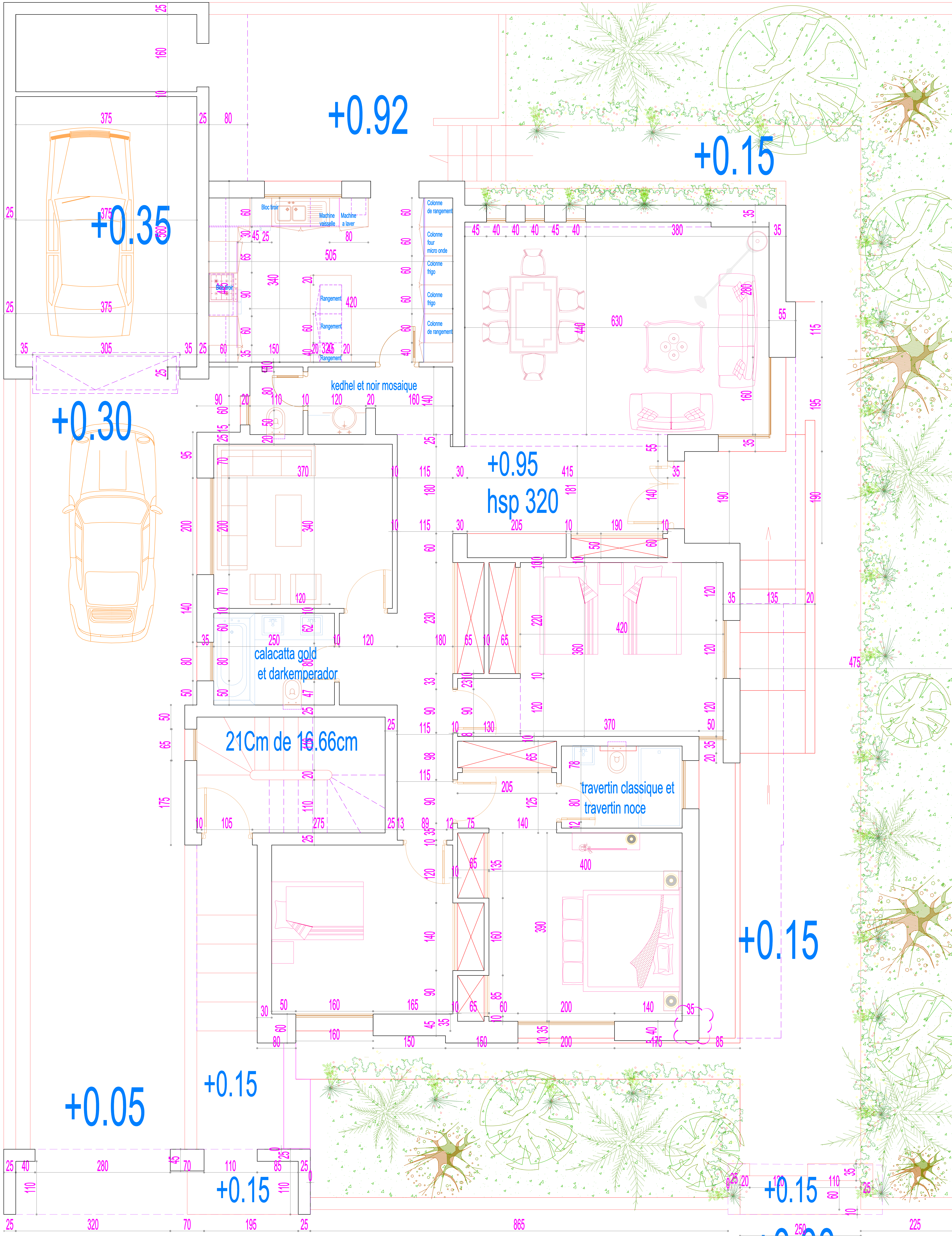
Plan Rdc 1ere tranche
